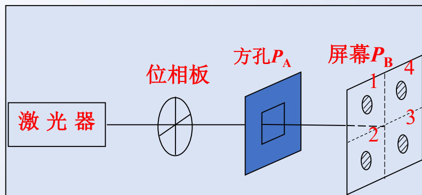
位相板法激光准直测量原理
